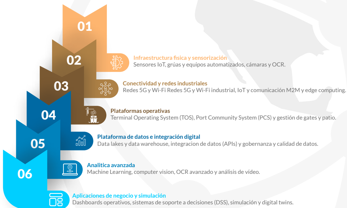
Figura 1. Capas de la arquitectura tecnológica
